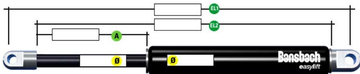
伸缩杆端连接件尺寸
